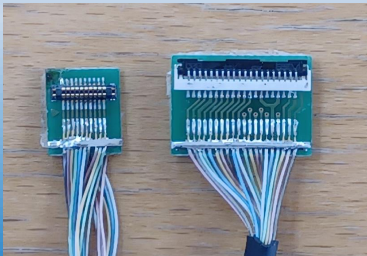
狭ピッチコネクタ—FPCコネクタ細線同軸ケーブル
