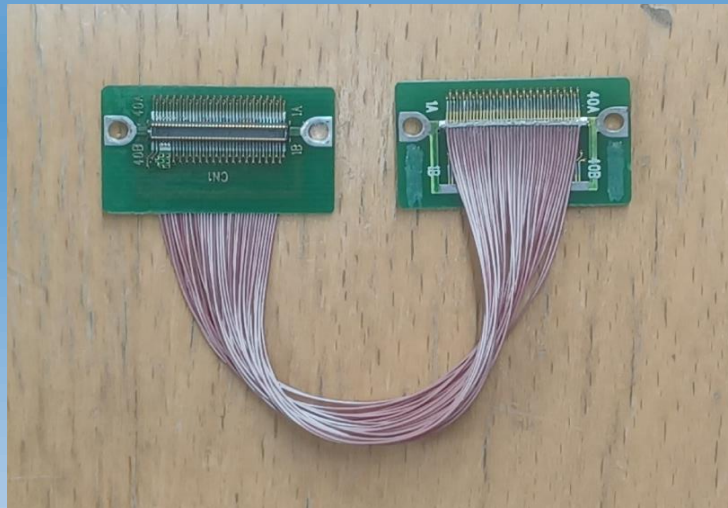
狭ピッチコネクタ細線同軸ケーブル
